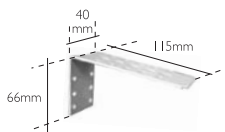
Escuadra de Extensión
